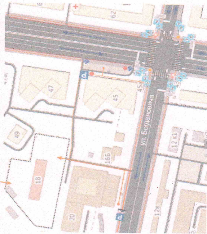
1.2. План-схема организации дорожного движения в непосредственной близости от МДОУ детского сада №40 с размещением соответствующих технических средств, маршруты движения обучающихся обучающихся и расположение парковочных мест
